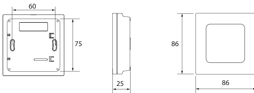
Prostorový termostat Danfoss Icon™ 088U1055
