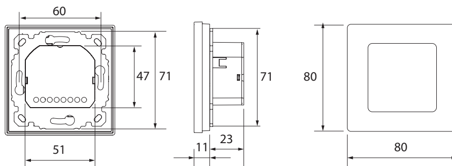
Prostorový termostat Danfoss Icon™ 088U1050
