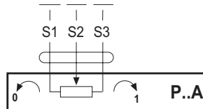
Schéma připojení
